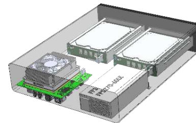
Smart IoT
